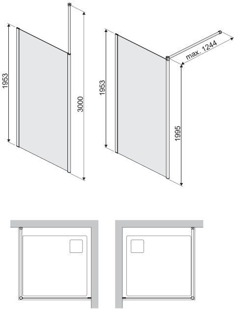
ECKVERSION, SEITENEINSTIEG / VERSION D'ANGLE, ENTRÉE PAR LE CÔTÉ / HOEKVERSIE, ZIJ-INSTAP
